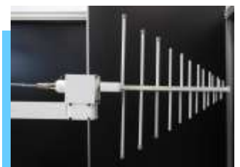
ギヤBOXを取付けることで、水平方向の偏波切 換が可能
